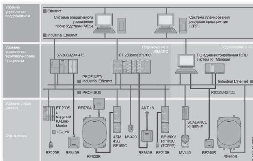
Пример интеграции RFID-систем в сеть автоматизации предприятия
